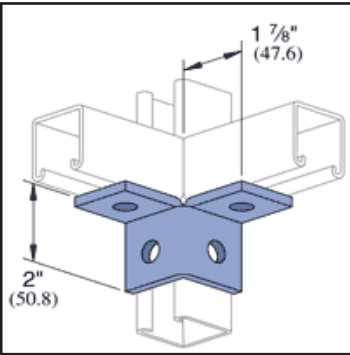
Codigo: CTLC-P2223
