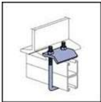
Codigo: CTLC-P2786
